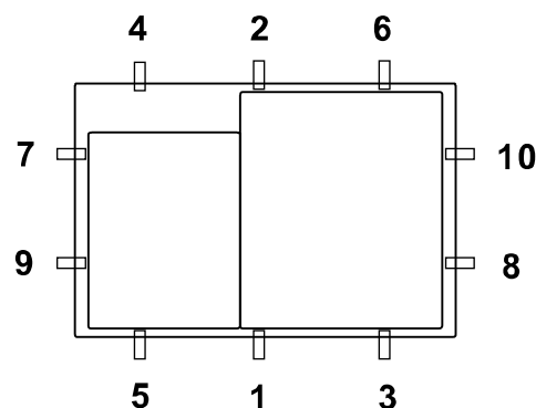
Secuencia de apriete de los clips
