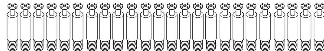
D Bolt M6 x 40mm QTY : 24 PCS
