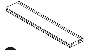
D 400*80*12mm(2pcs)
