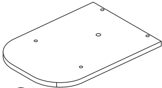
M 440*300*12mm(1pc)
