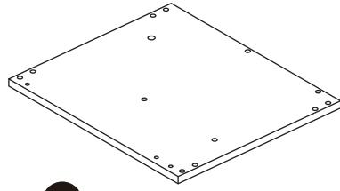
B 480*440*12mm(1pc)
