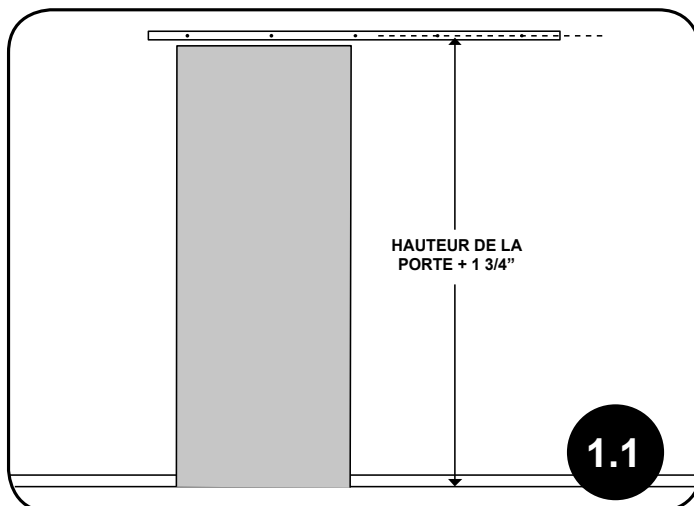
1. Installation du rail
