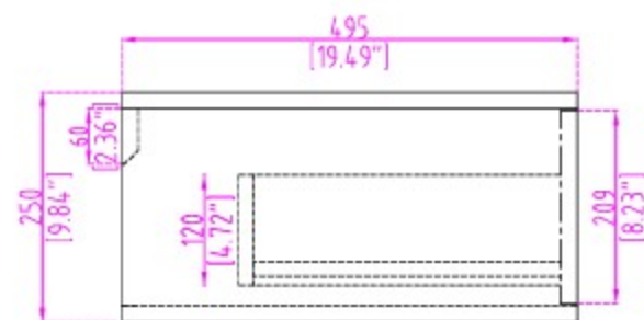
侧视图
