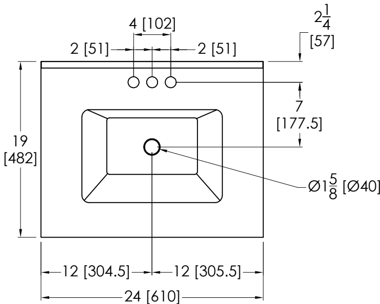
TOP / DESSUS / ARRIBA
