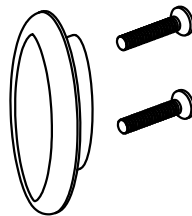
HANDLE M4 X 22mm QTY 2 SETS
