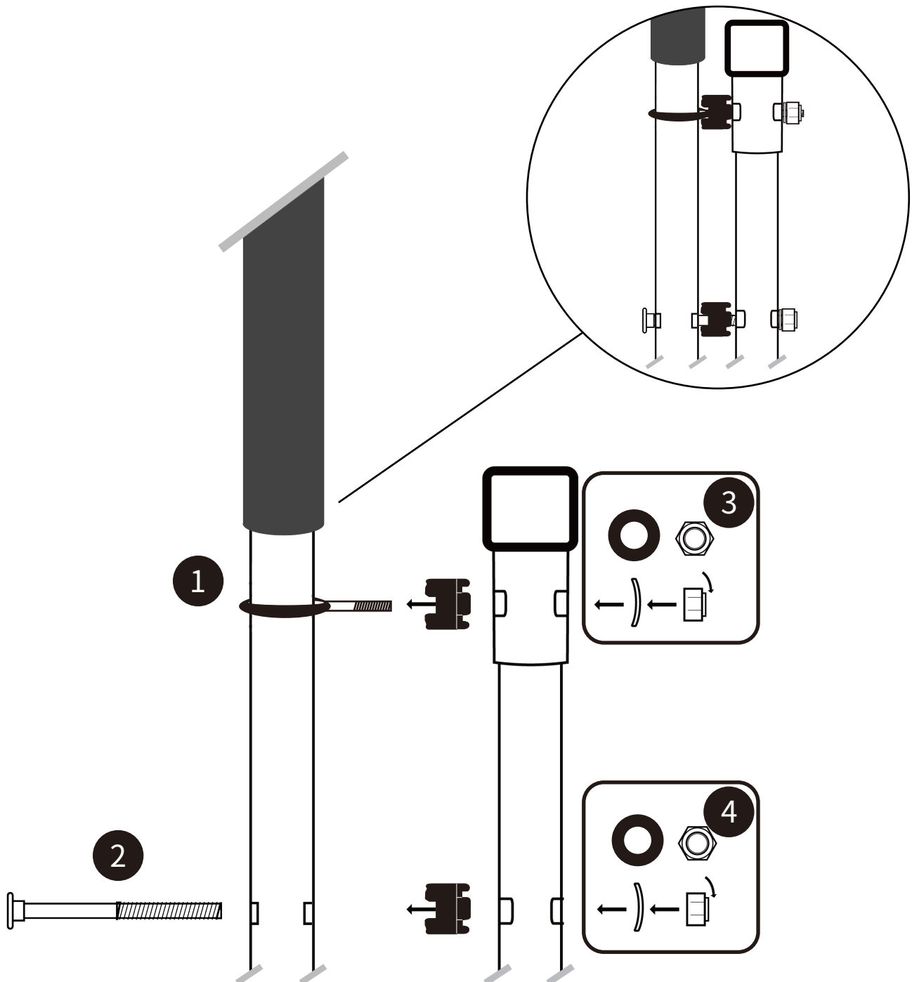
M6 X 85 mm Screw x 6
