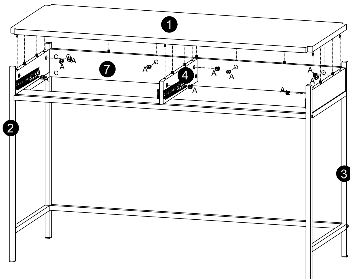
A.HIDDEN CAM - 10
