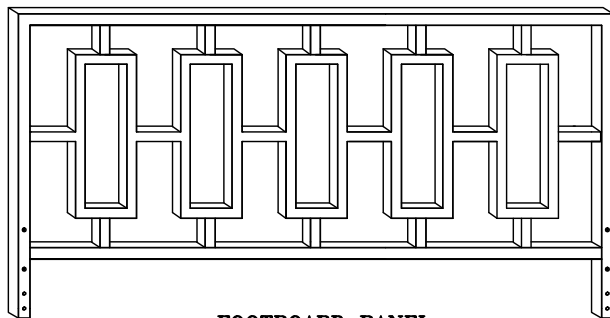
FOOTBOARD PANEL
