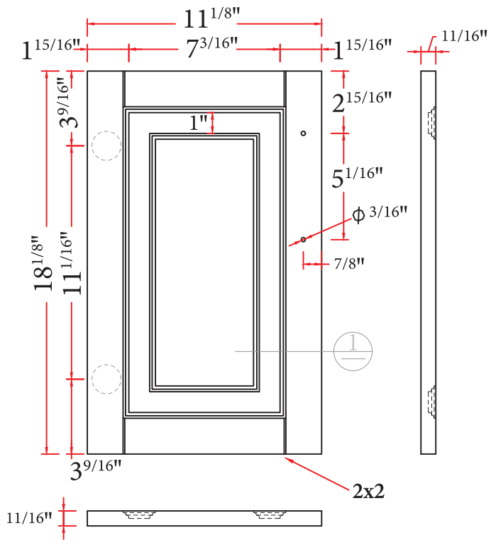
— DOOR —
