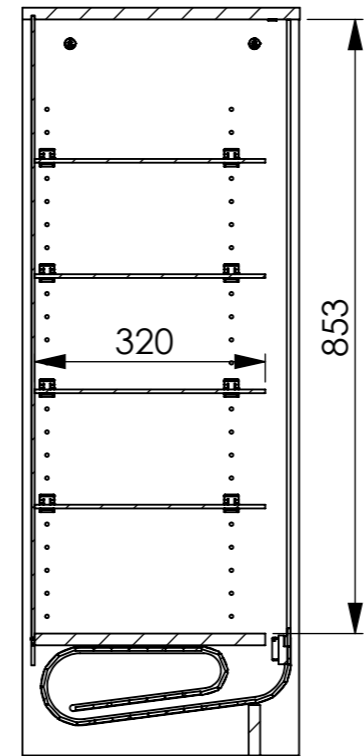
COUPE A-A ECHELLE 1 : 10.5
