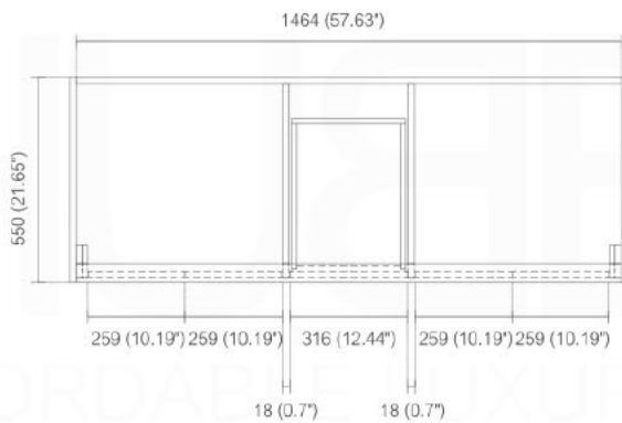
TOP ELEVATION
