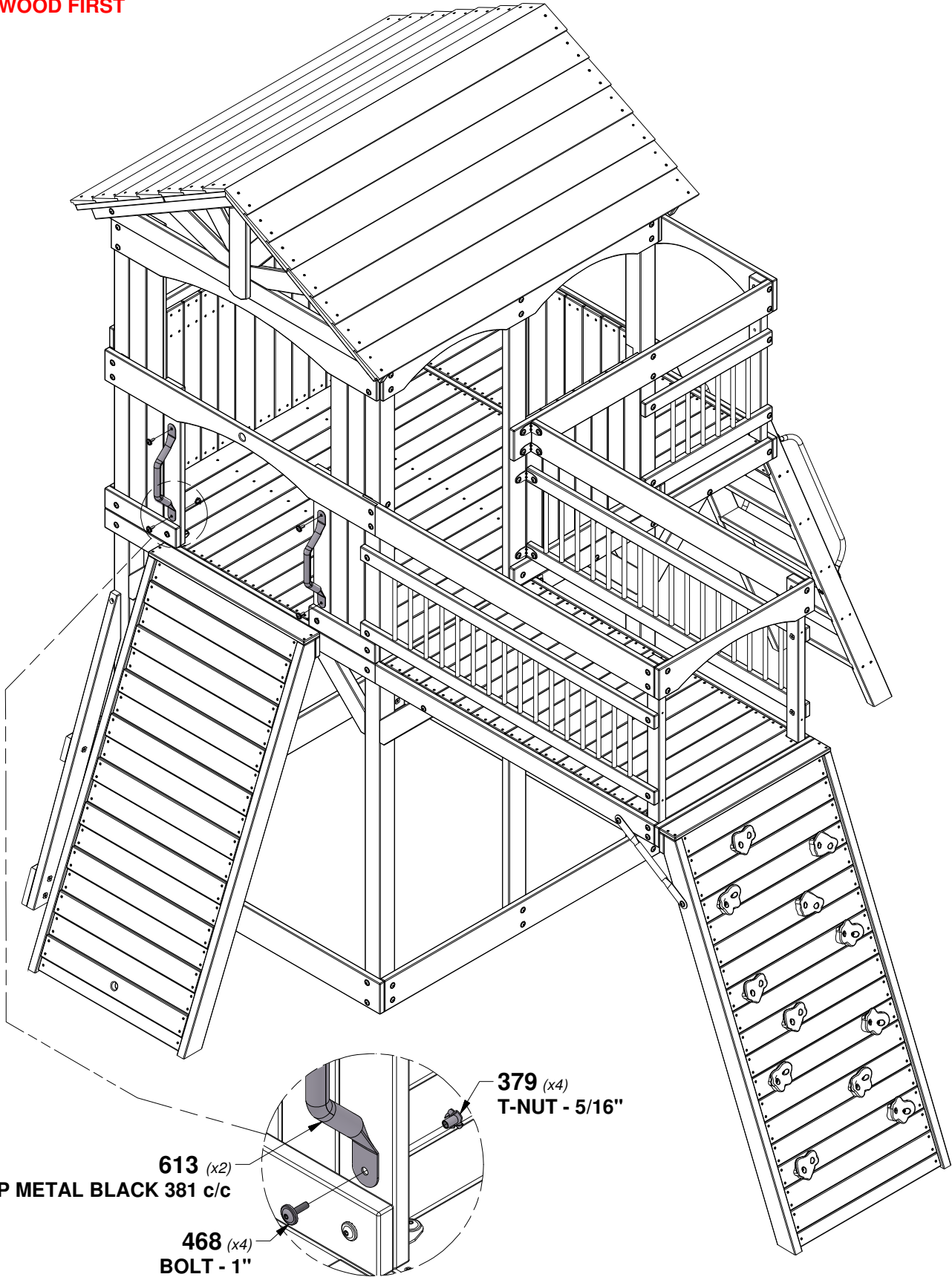
A4M00613 (x2) HAND GRIP METAL BLACK 381 c/c
