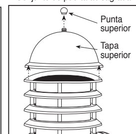
Figura 6 Unidades tipo lumbrera grande
