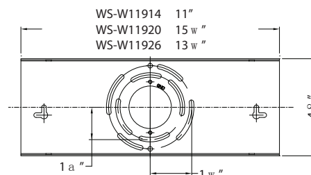
WS-W11914 & WS-W11920 & WS-W11926 Back Plate
