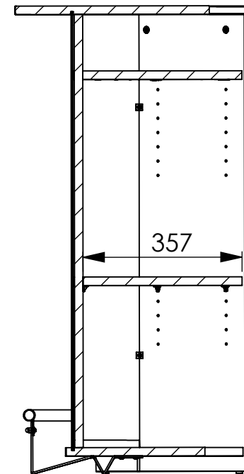
COUPE D-D ECHELLE 1 : 12
