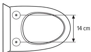
Distance requise entre Trous de fixation
