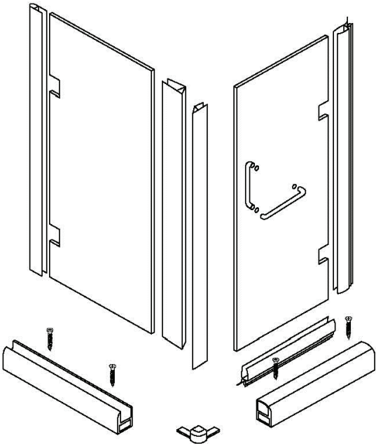
LEFT DOOR INSTALLATION
