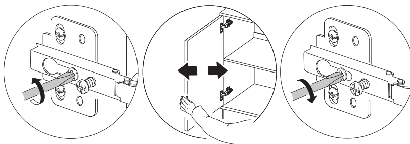
Adjust door depth
