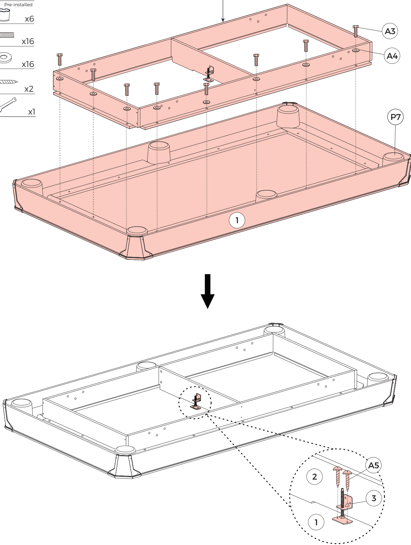
FIG. 3 Assembly / Ensamblaje FIG. 3 / FIG. 3 Assemblage
