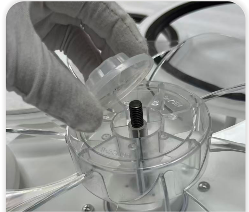
18 Attach the fan blade cap.
