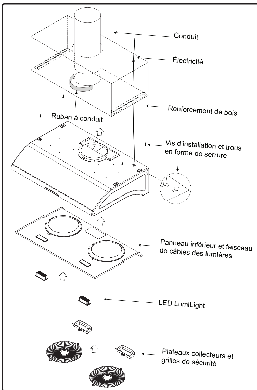
FIG. B
