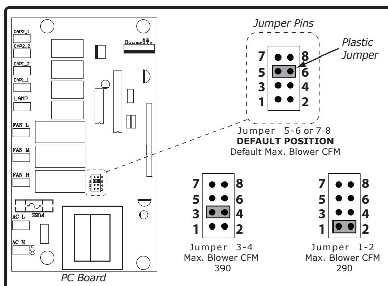
FIG. E
