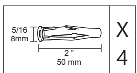
6 WALL ANCHOR CHAZO ANCLA
