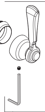
RP101323▲ Spout Flange & Gasket (1 Hole) Brida y Empaque (1 agujeros) Bride et Joint (1 trous)
