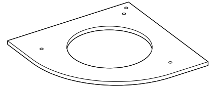
C 480*480*15mm(1pc)
