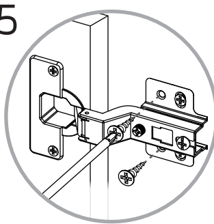
Hinge adjustment Ajuste de las bisagras
