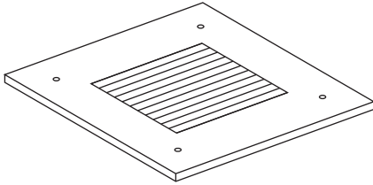
A 470*470*12mm(1pc)
