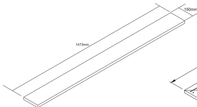
DESK TOP Qty:1
