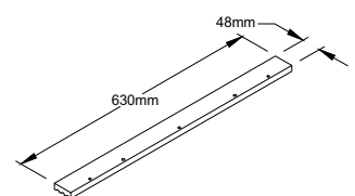
RAIL Qty:4
