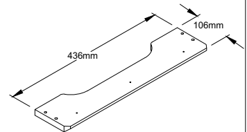
BOTTOM FRONT APRON Qty:2
