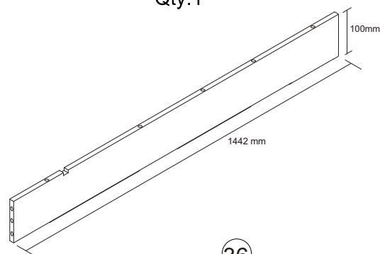
BACK PANEL Qty:1
