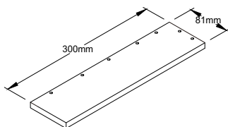
RIGHT DRAWER SIDE Qty:1
