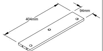
BOTTOM BACK APRON Qty:2
