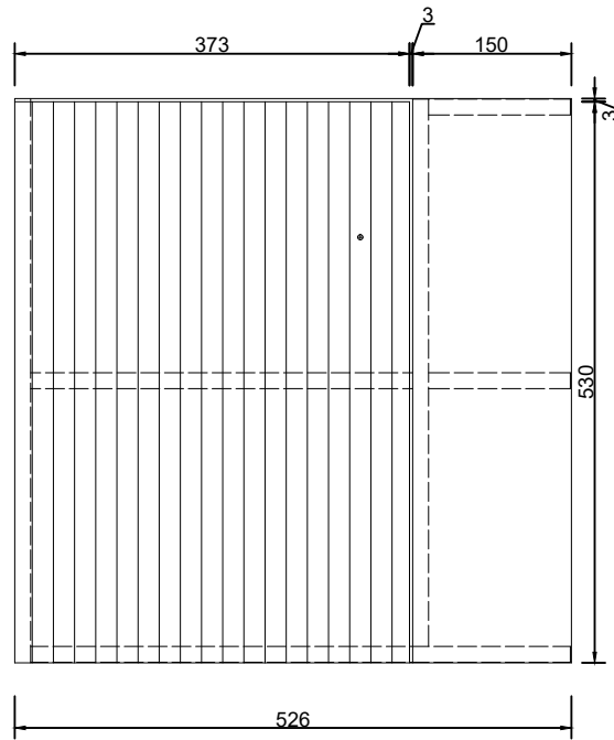
前视图
