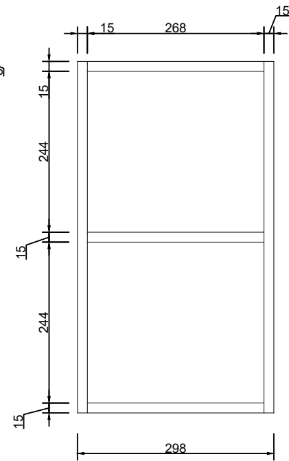
左视图
