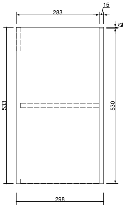
右视图
