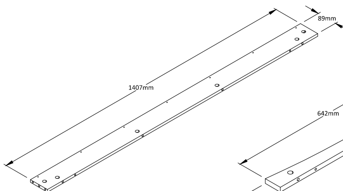
BACK RAIL Qty:2
