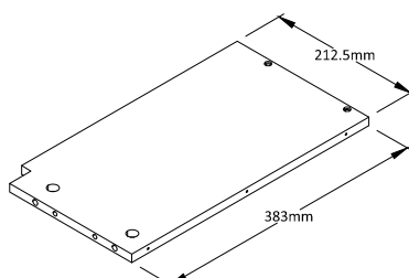
⑤⑩ UPPER LEFT BOTTOM Qty:1
