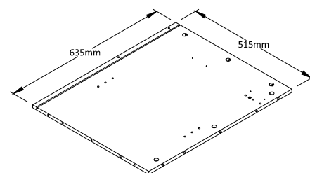
LEFT PARTITION Qty:1
