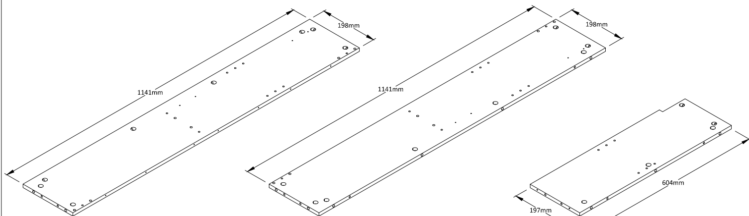
UPPER LEFT PANEL Qty:1
