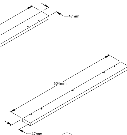
④⑧ UPPER RAIL Qty:2
