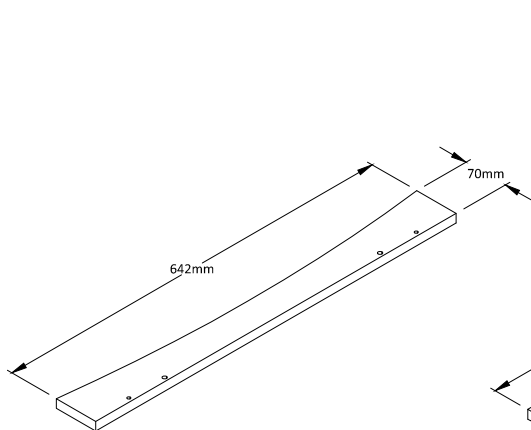
④⑥ RAIL Qty:1
