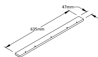
RAIL Qty:4
