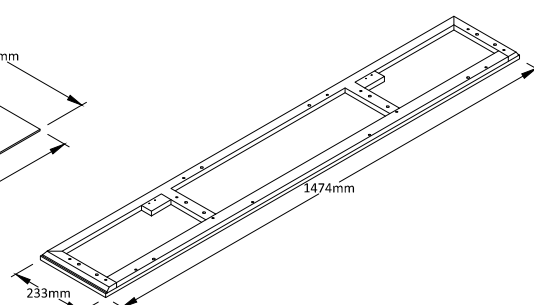
TOP Qty:1
