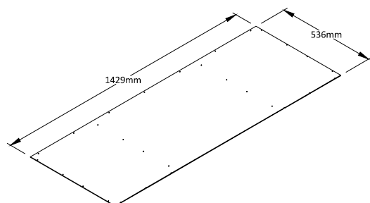
⑤② UPPER BACK PANEL Qty:1
