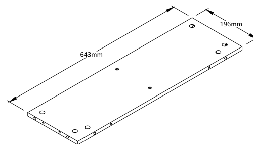
FIXED SHELF Qty:1
