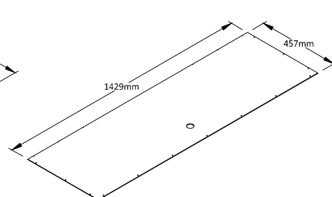
⑤④ UPPER BACK PANEL Qty:1
