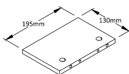
PARTITION Qty:1
