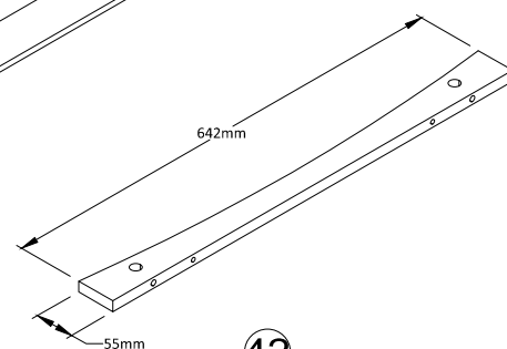
RAIL Qty:1
