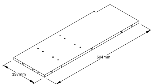
UPPER RIGHT PARTITION Qty:1
