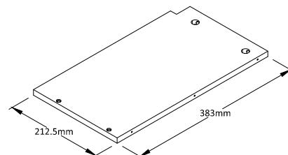
⑤① UPPER RIGHT BOTTOM Qty:1
