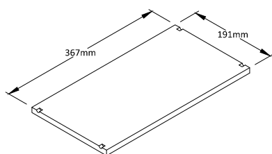
④⑨ ADJUSTABLE SHELF Qty:2
