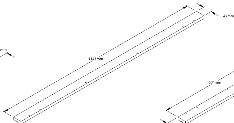
④⑦ UPPER RAIL Qty:2
