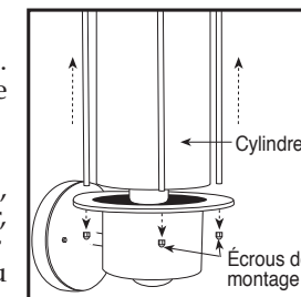
Figure 5 Appliques cylindriques
