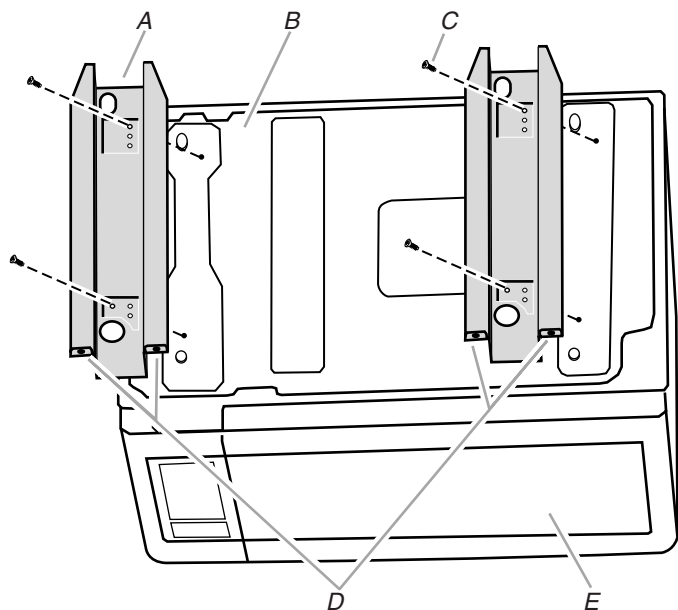
A. Tringles (2) B. Plancher du four à micro-ondes C. Vis courtes (4) D. Rebords E. Porte
