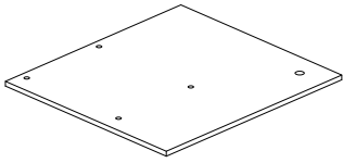
A 480*440*12mm(1pc)
