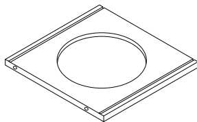
G 296*280*12mm(2pcs)
