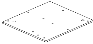
B 480*440*12mm(1pc)
