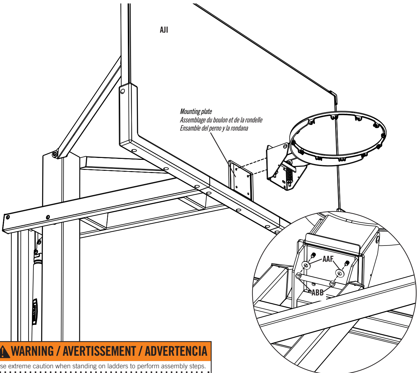
Rear view / Vue arrière / Vista posterior
