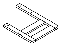
Side frame - shelf / Cadre latéral - étagère (1pc)
