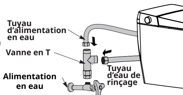
Tuyau d'alimentation en eau
