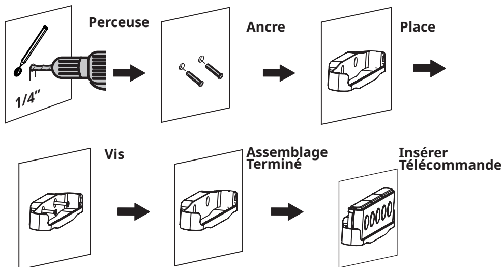
Perceuse et mèches *Non fournie
