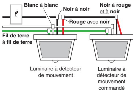
Raccordement d'un luminaire à détecteur de mouvement pour la commande d'un autre luminaire à détecteur de mouvement
