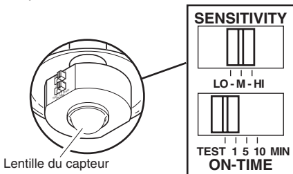
Lentille du capteur
