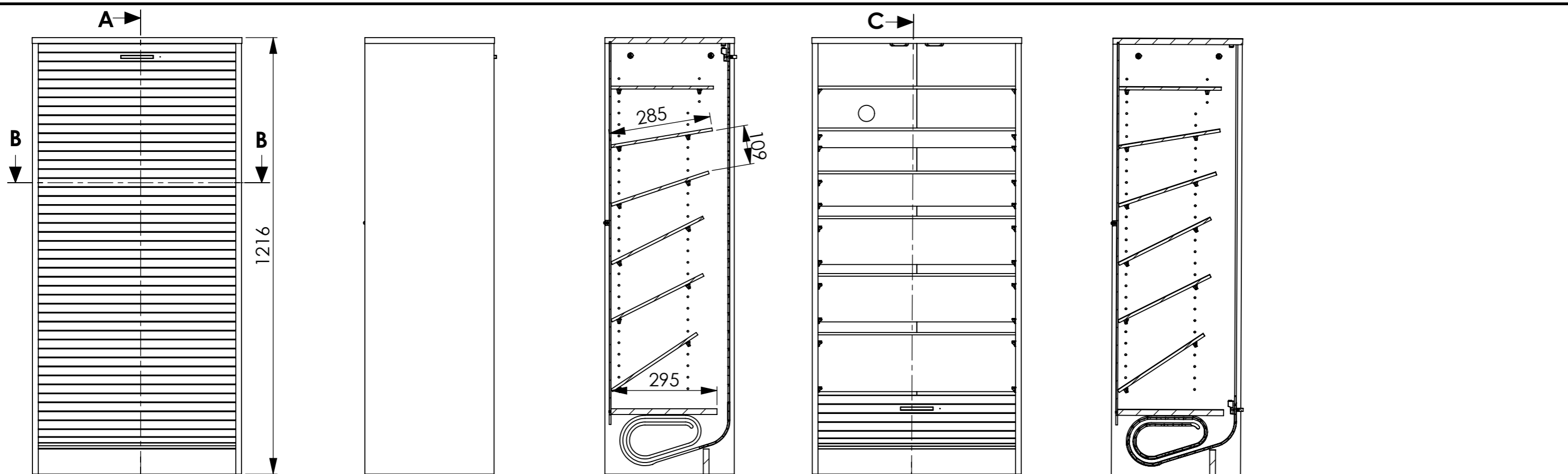
COUPE A-A ECHELLE 1 : 11
