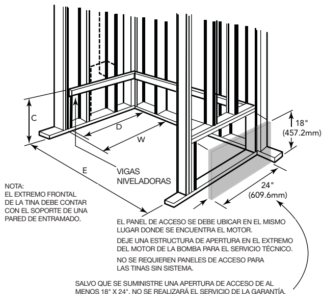
IMAGEN 2 INSTALACIÓN TÍPICA EN NICHOS
