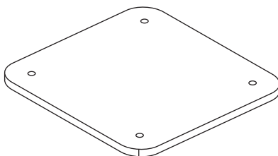
B 400*400*12mm(1pc)
