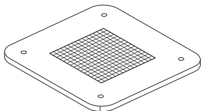
A 400*400*12mm(1pc)
