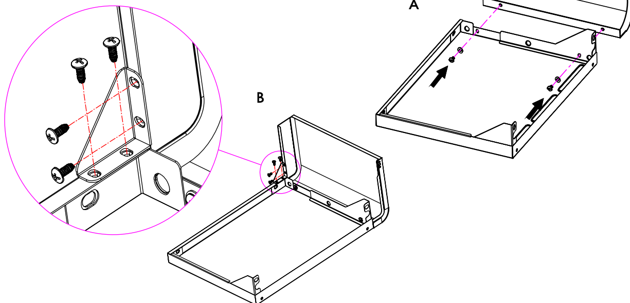
Rondelle plate M5 Qté : 2 pièces
