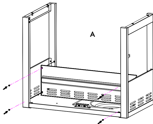
Assemblage du panneau droit
