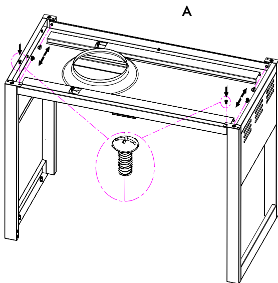
Tornillo M6x13 Cantidad: 4 piezas
