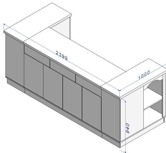
全视图
