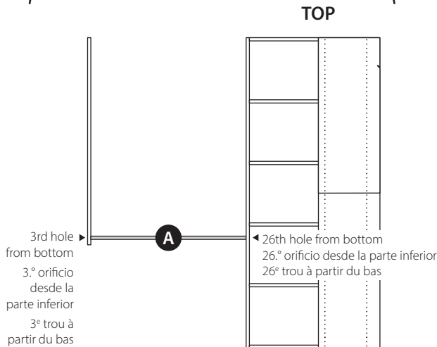
BOTTOM
