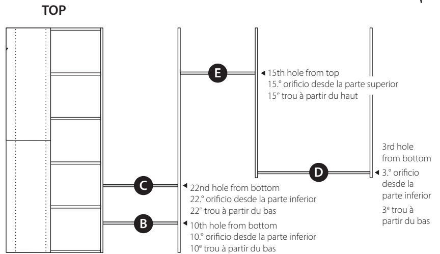
BOTTOM
