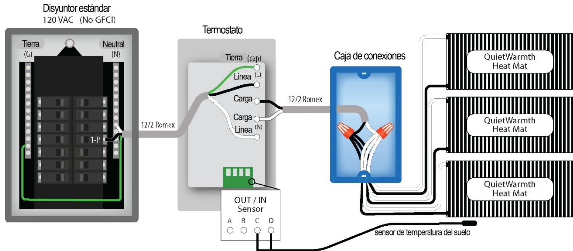
DIAGRAMA TÍPICO DE CABLEADO ELÉCTRICO DE 120V
