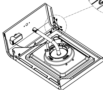
Rondelle plate M5 Qté : 2 pcs
