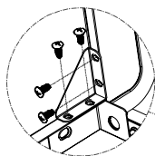
Tornillo M6x13 Cantidad: 4 piezas
