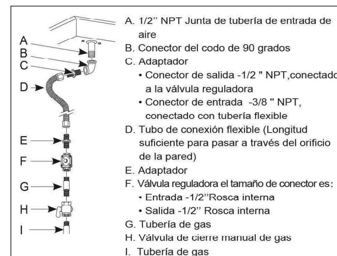
Instalación sugerida cuando no hay interferencias debajo de la estufa
