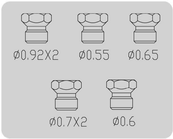
液化石油气转换套件
