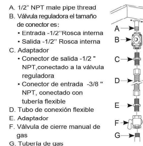
Instalación sugerida para evitar interferencias debajo de la estufa
