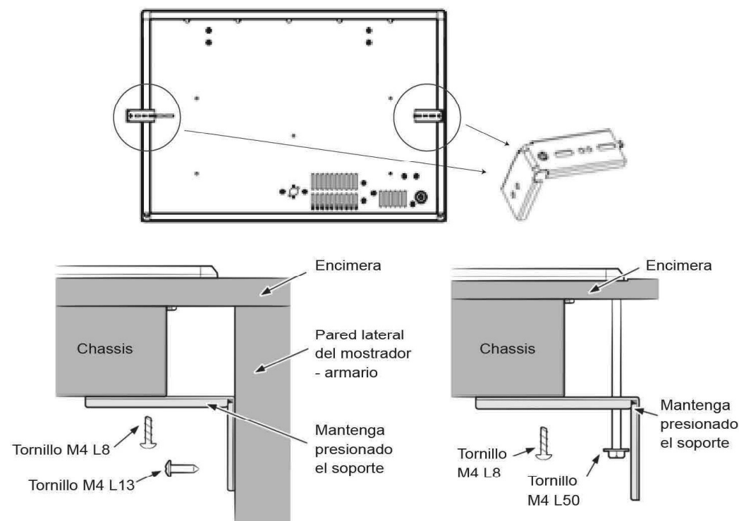
métodos de instalación 1
