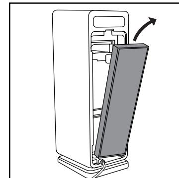
b. Retirez la combinaison de filtres de l'appareil. Remarque : le préfiltre et le filtre au charbon sont combinés en un seul filtre qui s'accroche au filtre HEPA par une bande Velcro.
