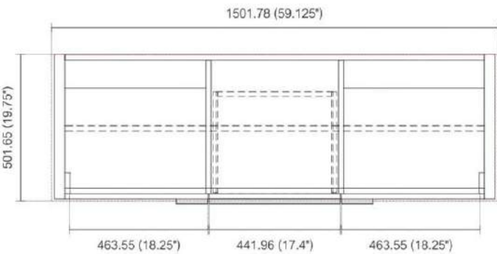
. TOP ELEVATION
