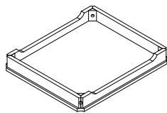
Bottom Frame Cadre inférieur
